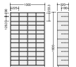
■24人用 SBM-46 ¥315,900◎ 外寸法/W1000×D320×H1600 4列6段 質量:53kg
