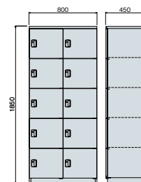
A112-01
