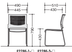
E278F-1-□ E278F-3-□
