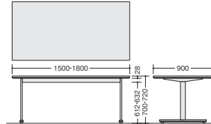
KG11890C-□、KG11590C-□ ノックダウン式③ KGTH1890C-□、KGTH1590C-□
