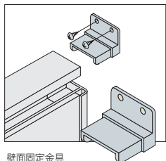
壁面固定金具 (ローパーティション(BP型))
