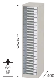
KCT2601-AW ¥53,600 外寸法 / W277×D400×H1200 引出し内寸法 / W226×D308×H36 1列浅型26段A4用 質量:23kg
