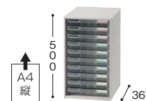
KCT110TR-AW ¥17,600 外寸法 / W275×D367×H500 引出し内寸法 / W242×D340×H40 1列10段A4用 質量:8kg
