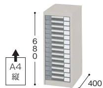
KCT1401-AW ¥38,900 外寸法 / W277×D400×H680 引出し内寸法 / W226×D308×H36 1列浅型14段A4用 質量:13.9kg
