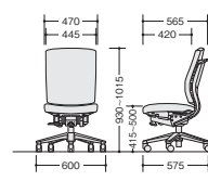
FEN512-□
